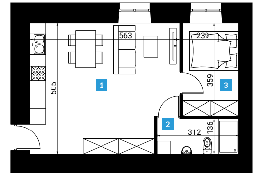
Rzut lokalu
