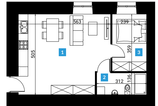
Rzut lokalu
