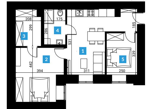
Rzut lokalu
