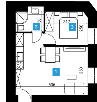
Rzut lokalu M47
