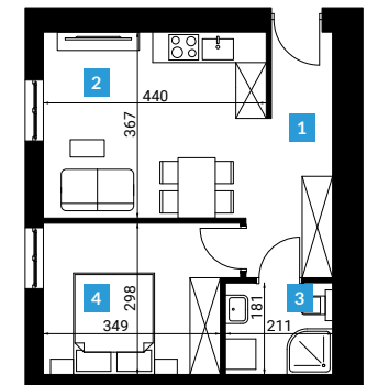
Rzut lokalu M51
