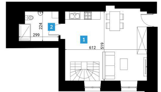
Rzut lokalu
