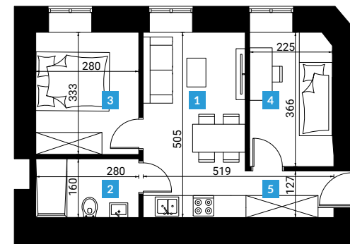
Rzut lokalu
