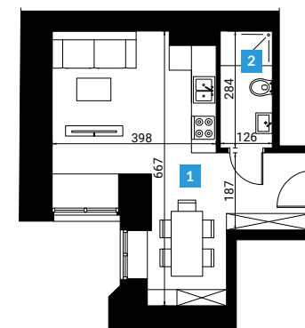
Rzut lokalu
